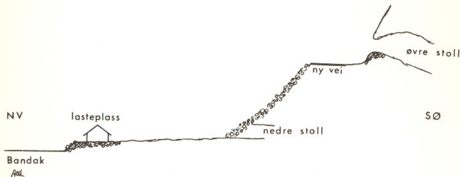
Skisse over nedre del av Tveitsto flusspatgruve.
