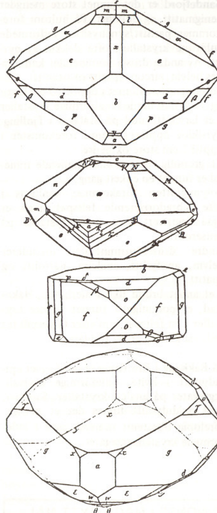
Ditolitt – Tafjordtunnelen (over).
