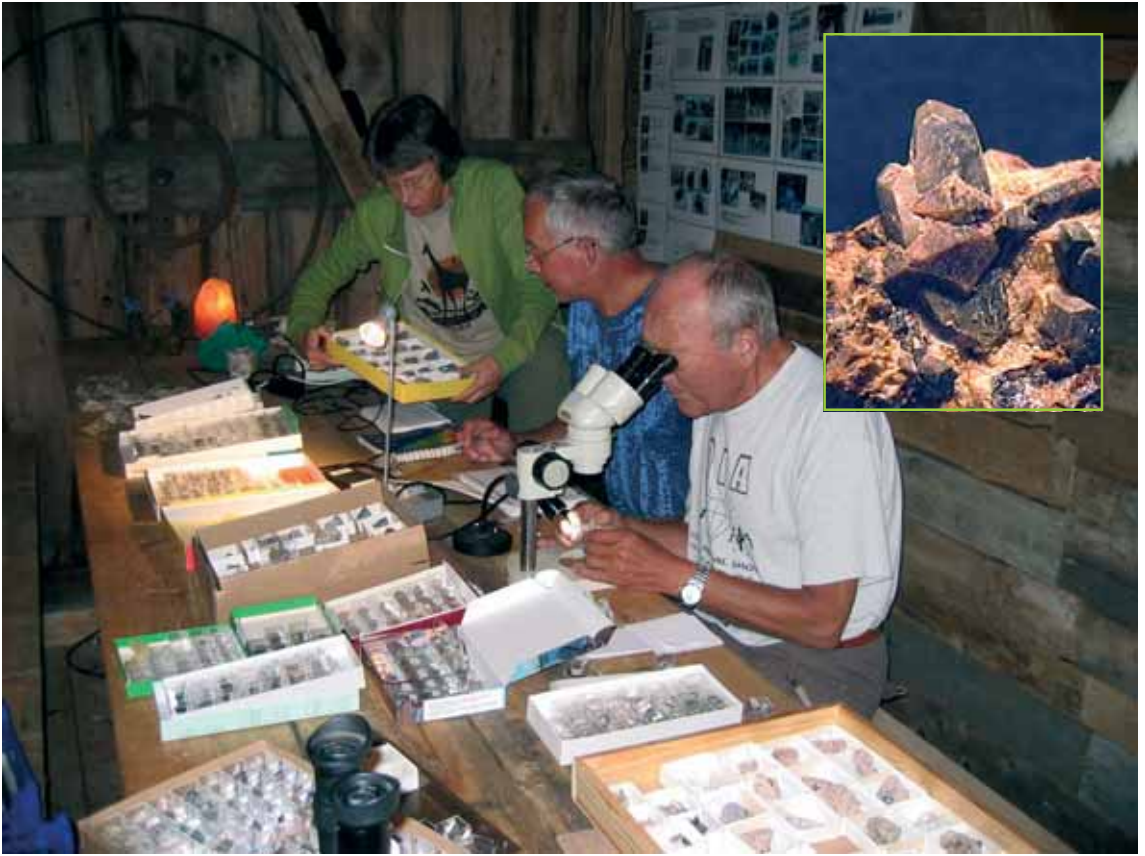
Innfelt: Xenotim og zirkon.
