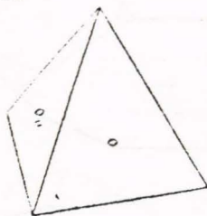
Tritomitt
