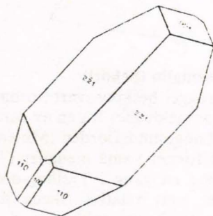
Titanitt
