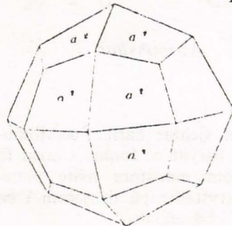
Analcim
