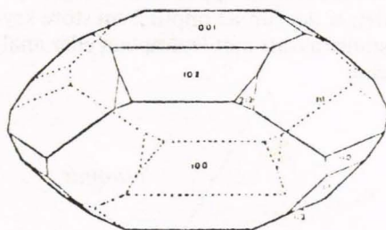
Titanitt
